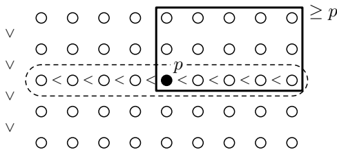
Obrázek 10.9: Pětky a jejich mediány
