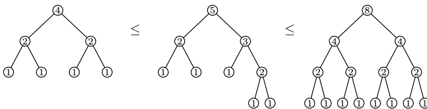
Obrázek 10.6: Obecné n jsme sevřeli mezi n^- a n^+
