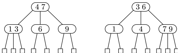
Obrázek 8.7: Dva (2,3)-stromy pro tutěz množinu klíčů
