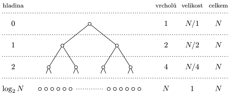
Obrázek 10.3: Strom rekurze algoritmu MERGESORT
