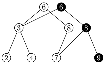
Obrázek 16.12: Vložení prvku 9 do persistentního stromu
