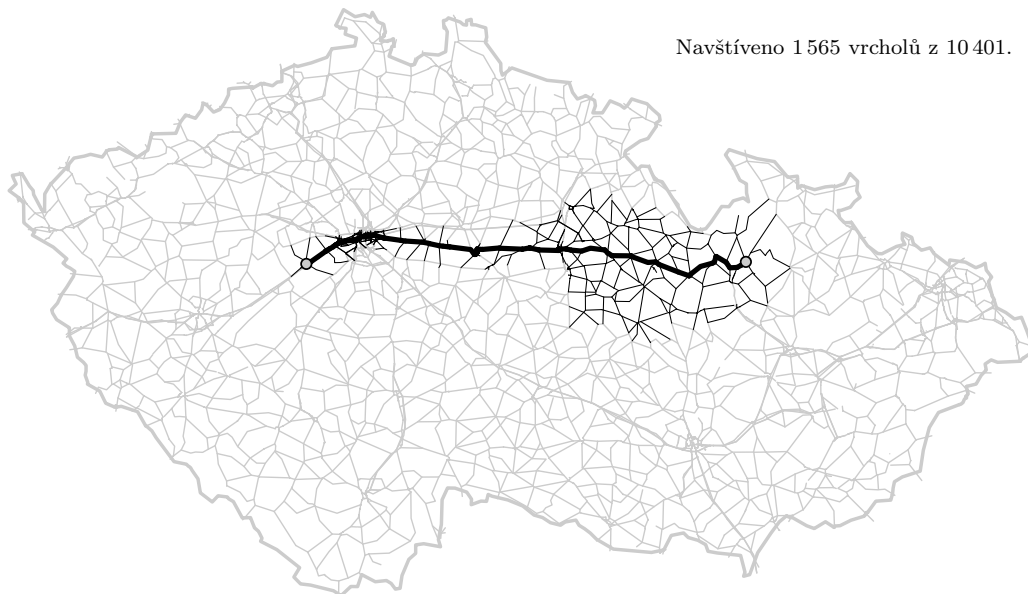
Obrázek 6.6: Hledání v mapě obousměrným algoritmem A*
