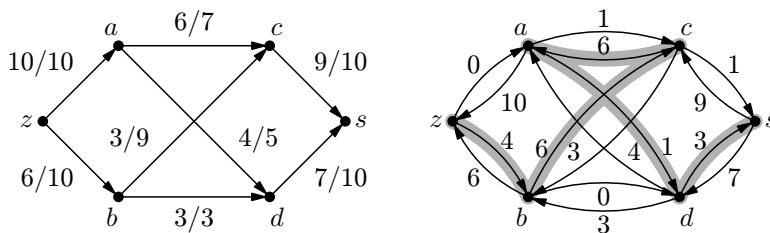
Obrázek 14.4: Fordův-Fulkersonův algoritmus v řeči rezerv: vlevo tok/kapacita, vpravo rezervy a nenasycená cesta
