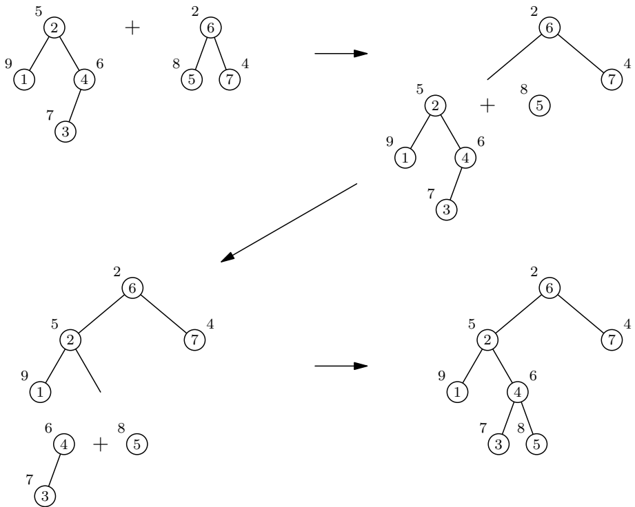
Obrázek 11.4: Spojení dvou treapů.
