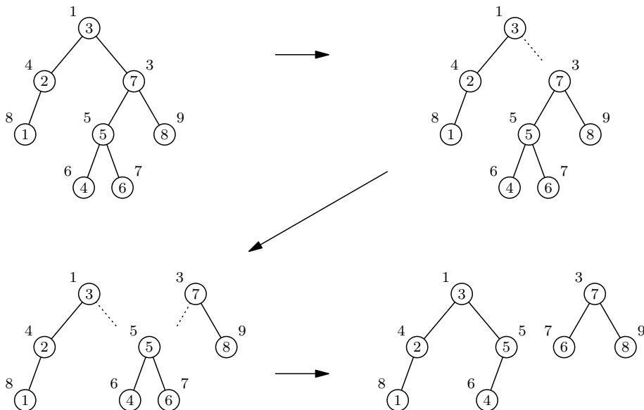
Obrázek 11.5: Rozdělení treapu podle x = 5 .
