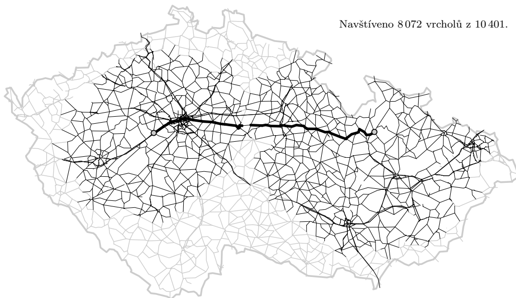
Obrázek 6.4: Hledání v mapě obousměrným Dijkstrůvým algoritmem
