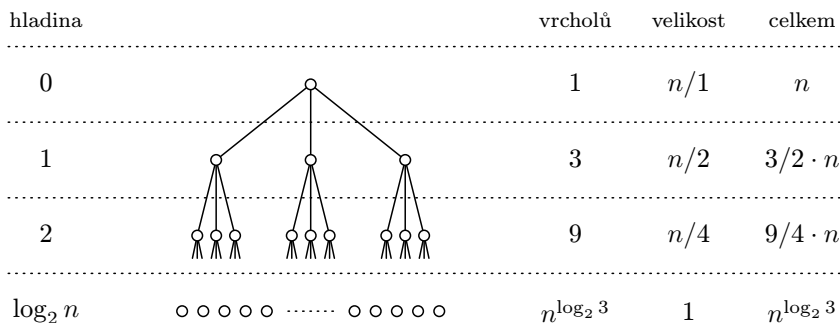
Obrázek 10.5: Strom rekurze algoritmu NÁSOS
