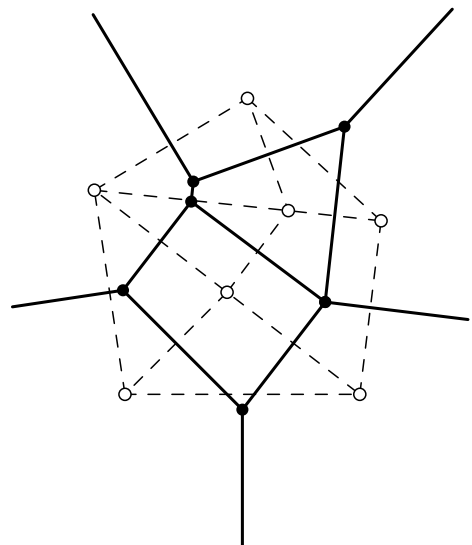
Obrázek 16.7: Voroného diagram
