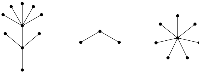
Obrázek A.5: Les složený ze tří stromů
