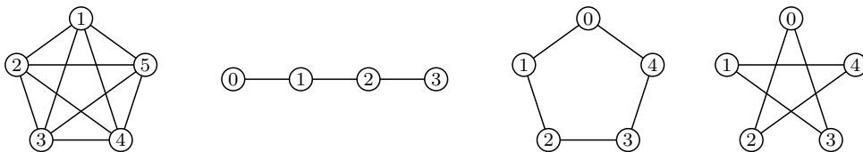
Obrázek A.1: Grafy K_5 , P_3 , C_5 a \overline{C_5}
