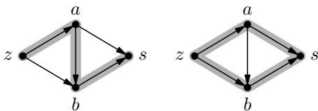
Obrázek 14.3: Algoritmus v úzkých (všude c = 1 )
