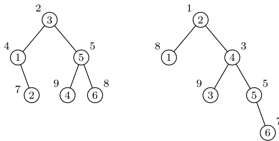
Obrázek 11.3: Dva různé treapy se stejnými klíči a různými prioritami. Čísla uvnitř vrcholů jsou klíče, čísla vně vrcholů priority.
