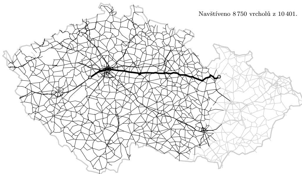
Obrázek 6.3: Hledání v mapě Dijkstrovým algoritmem
