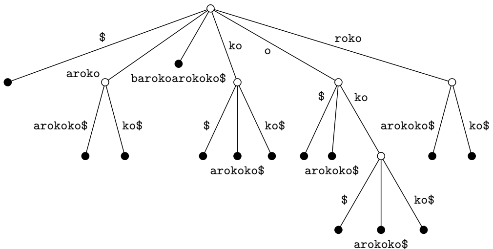
Obrázek 13.4: Suffixový strom pro slovo barokoarokoko
