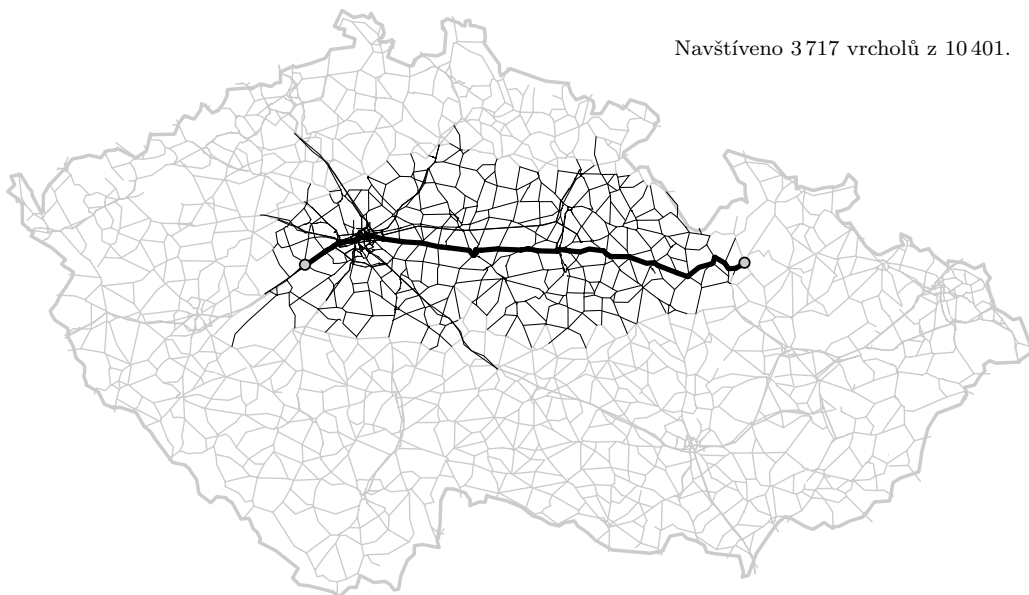
Obrázek 6.5: Hledání v mapě algoritmem A*
