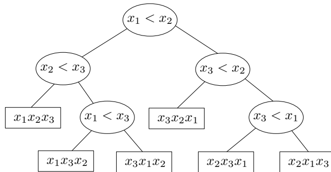
Obrázek 3.1: Příklad rozhodovacího stromu pro 3 různé prvky
