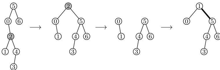
Obrázek 9.7: Postup mazání ze splay-stromu
