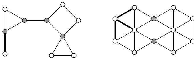
Obrázek A.6: Nalevo mosty a artikulace, napravo vrcholový řez velikosti 2 a hranový řez velikosti 3
