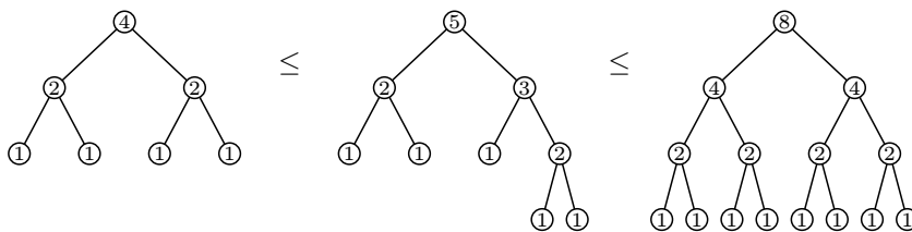
Obrázek 10.6: Obecně n jsme sevřeli mezi n^- a n^+
