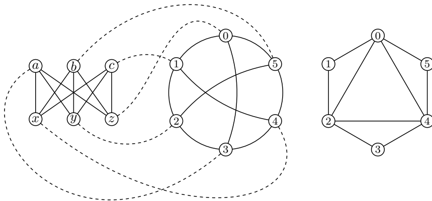
Obrázek A.3: První dva grafy jsou izomorfní, třetí s nimi izomorfní není.
