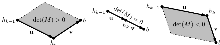
Obrázek 16.4: Jak vypadají determinanty různých znamének v rovině
