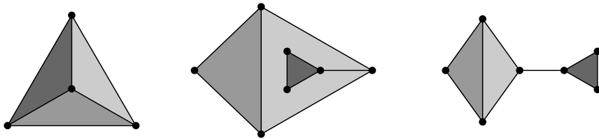
Obrázek A.7: Grafy nakreslené do roviny. Šedé jsou vnitřní stěny, bílá stěna vnější.
